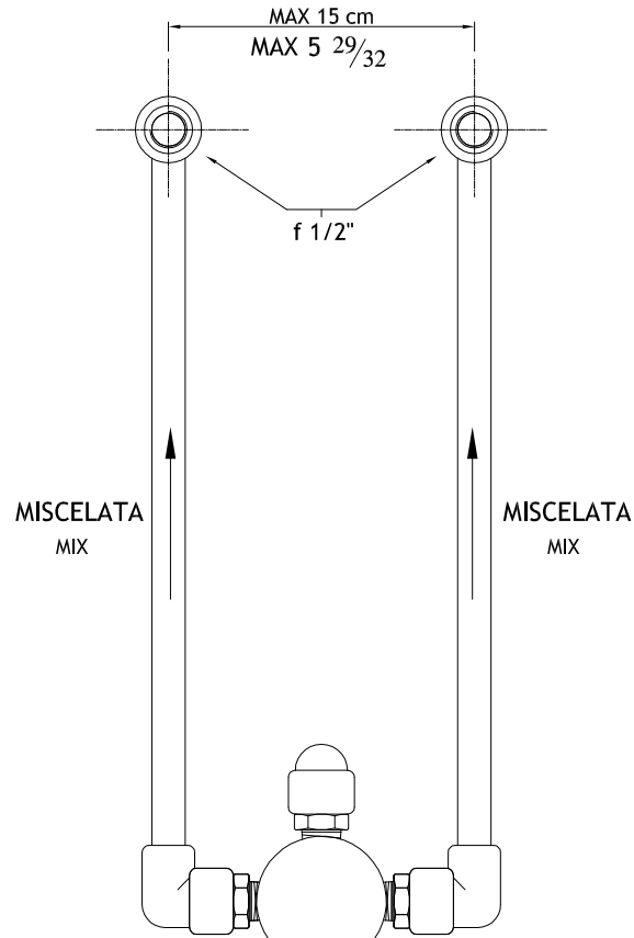
INDICAZIONI PER IL RIVESTIMENTO DETAILS FOR WALL COVERING
